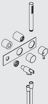
E0BA0468ECINOX
