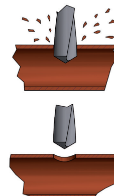
Foratura Drilling
